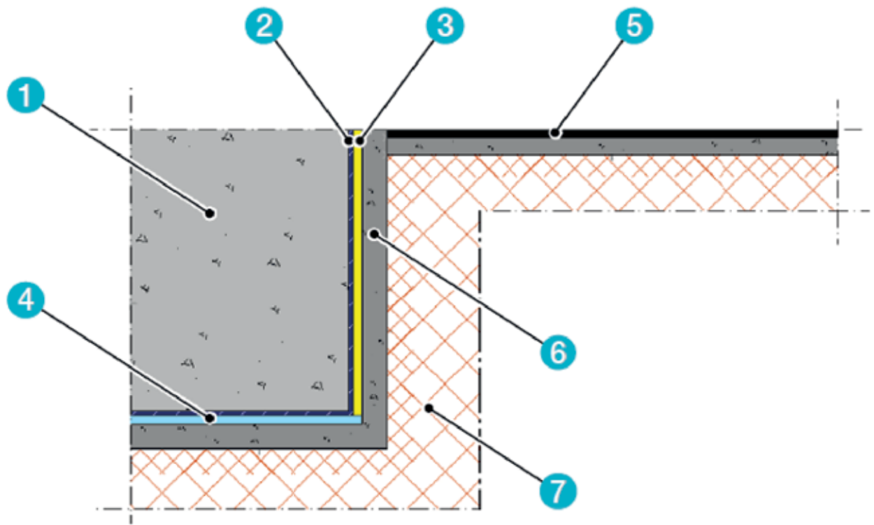
Figura 4-5. Aislante basamento (ejemplo).
