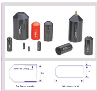
Capuchones termoretráctiles con o sin válvula de alivio
